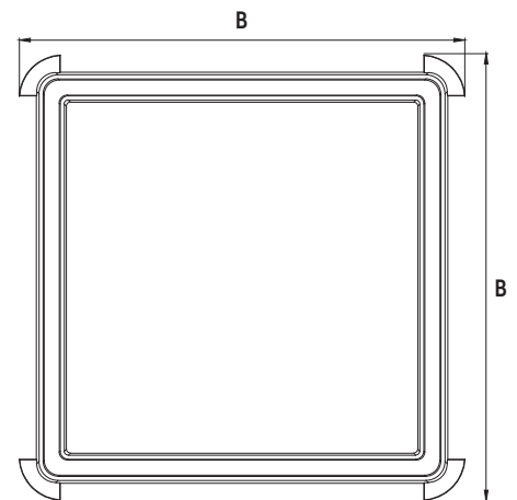
SECCIÓN MARCO
