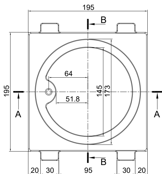
MARCO VISTA SUPERIOR
