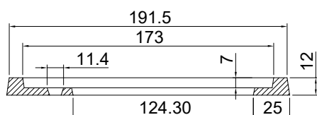
SECCIÓN MARCO A-A
