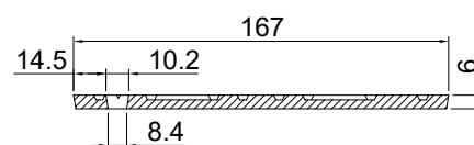
SECCIÓN TAPA C-C
