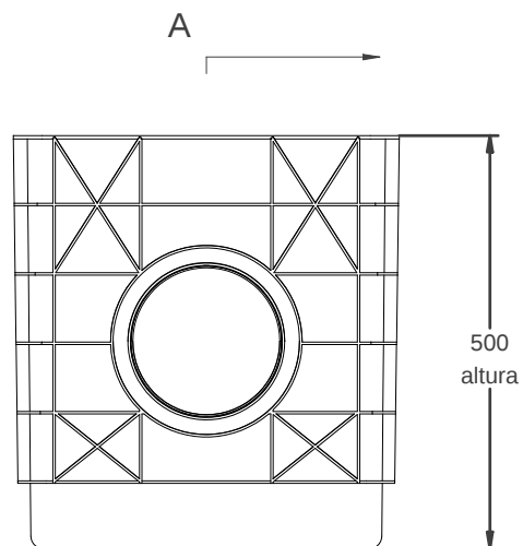
A vista alzado 1:10
