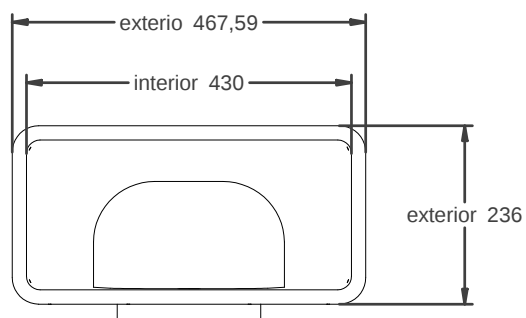
vista en planta 1:10
