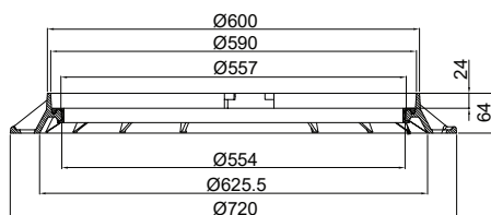
SECCIÓN MARCO
