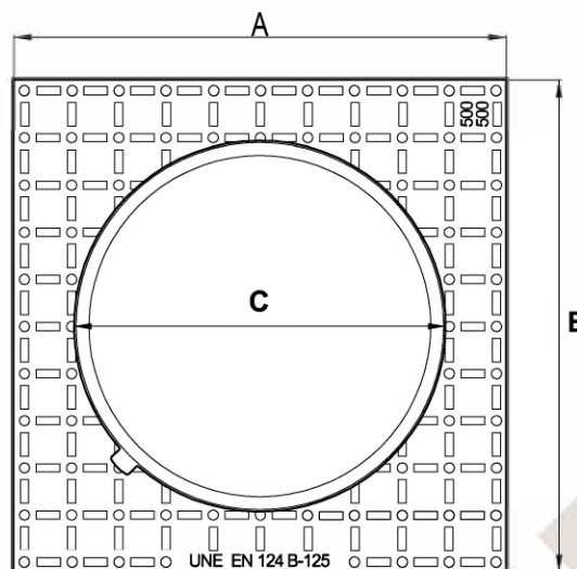
TAPA. VISTA SUPERIOR.
